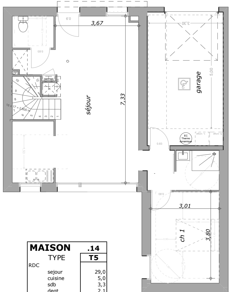
PLAN RDC
