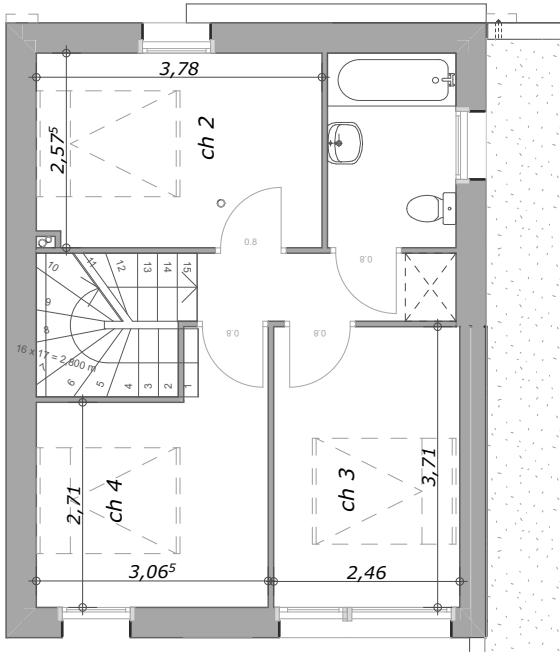
PLAN ETAGE
